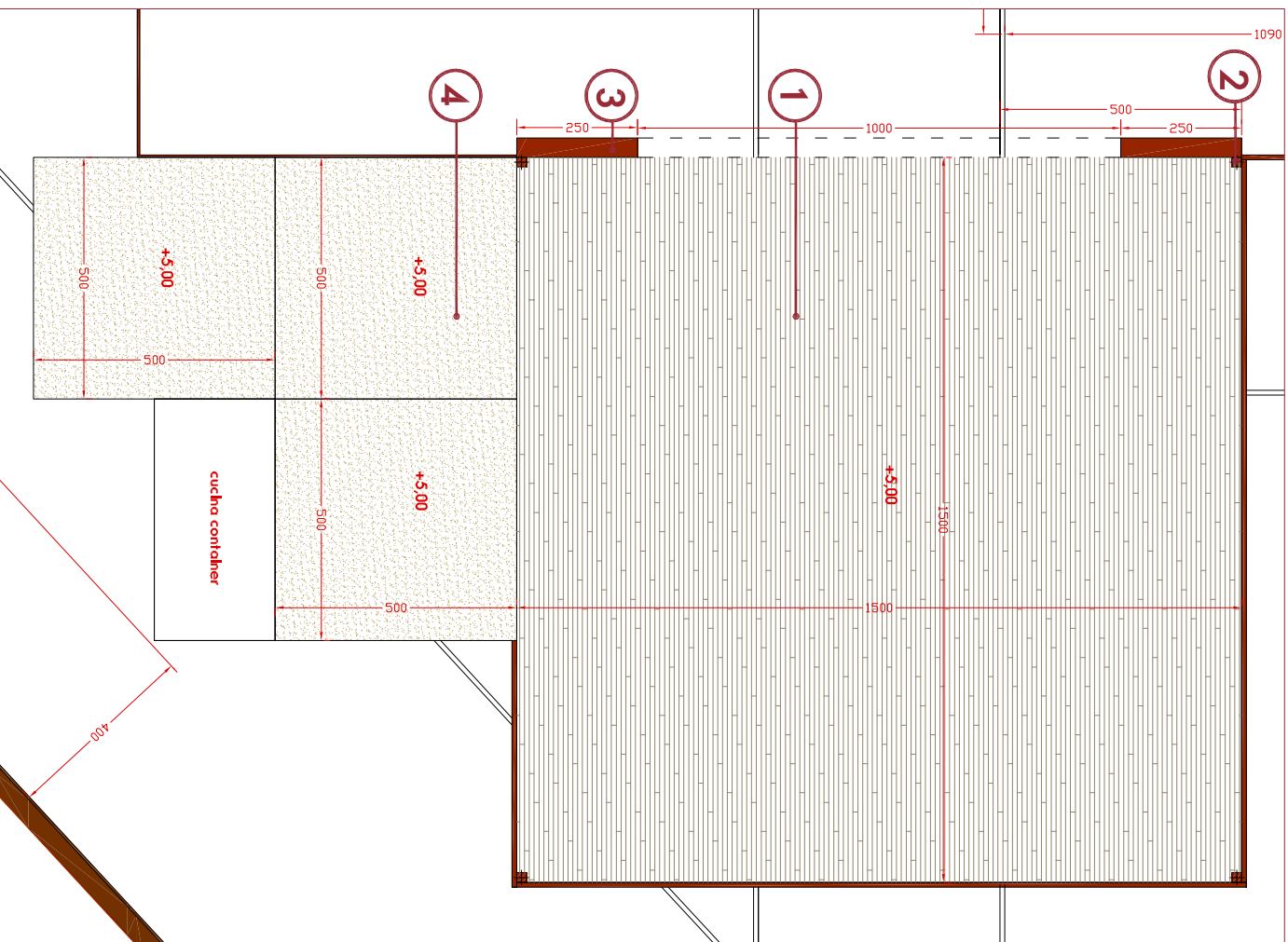
Planimetria
