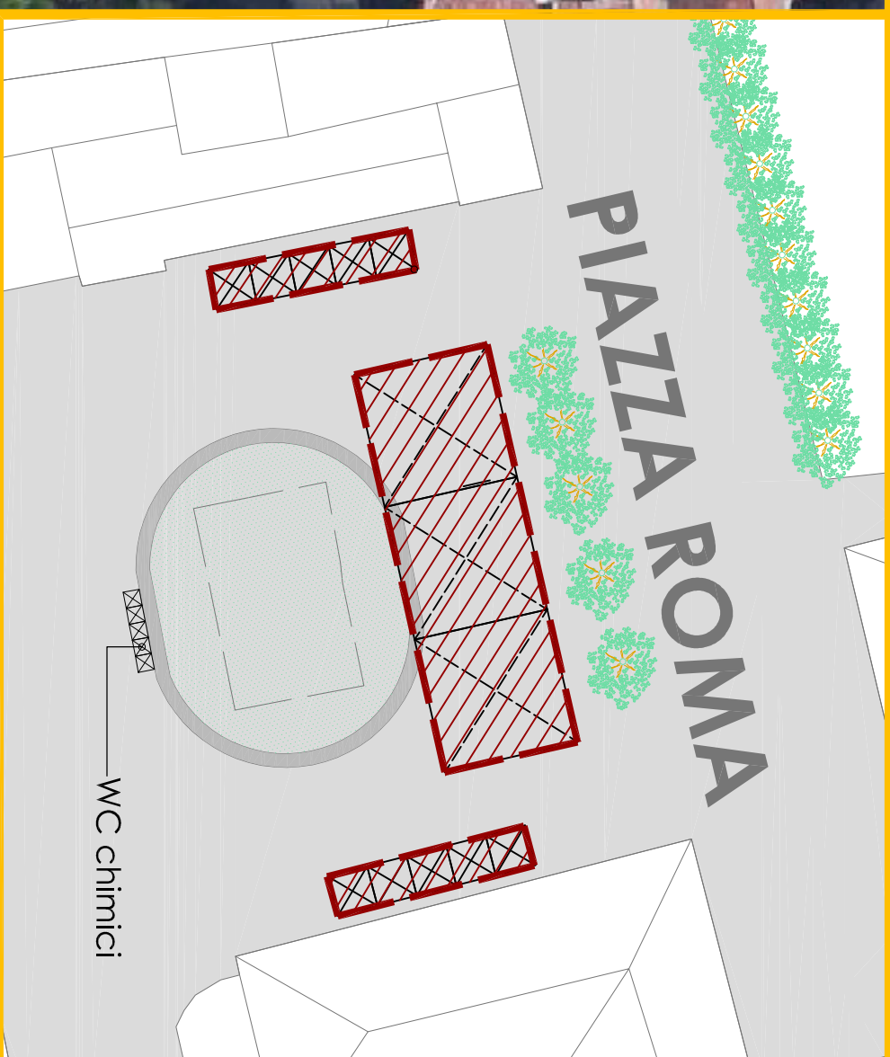
Planimetria scala 1:500
